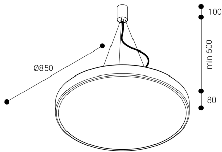
Dimensiones (mm):
