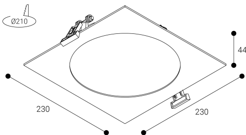
Dimensiones (mm):
