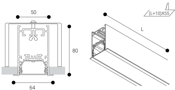
Dimensiones (mm):
