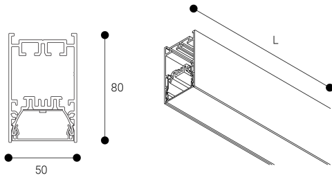
Dimensiones (mm):
