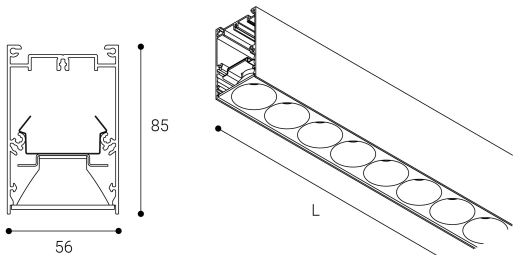
Dimensiones (mm):
